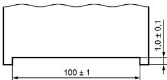
Рисунок 9 - Схема аппликатора для нанесения клея
